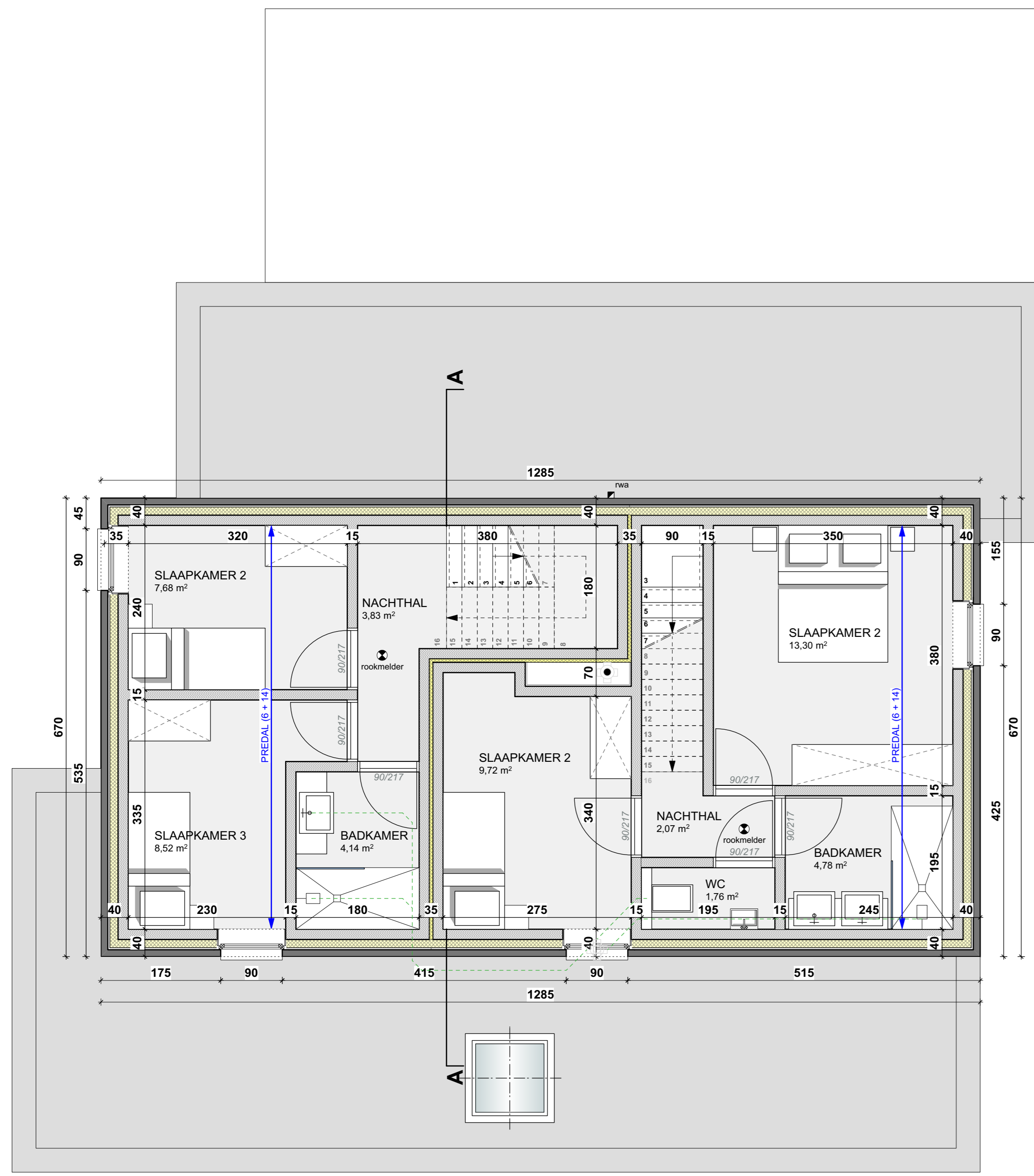
VERDIEPING 2 BLOK A schaal 1/50
