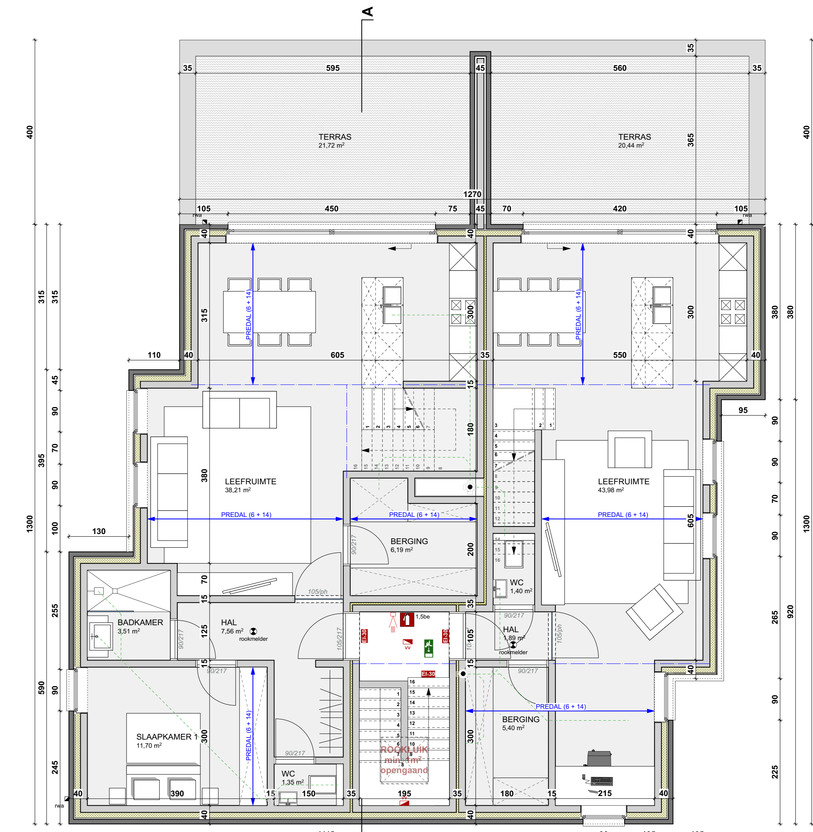
VERDIEPING 1 BLOK C schaal 1/50
