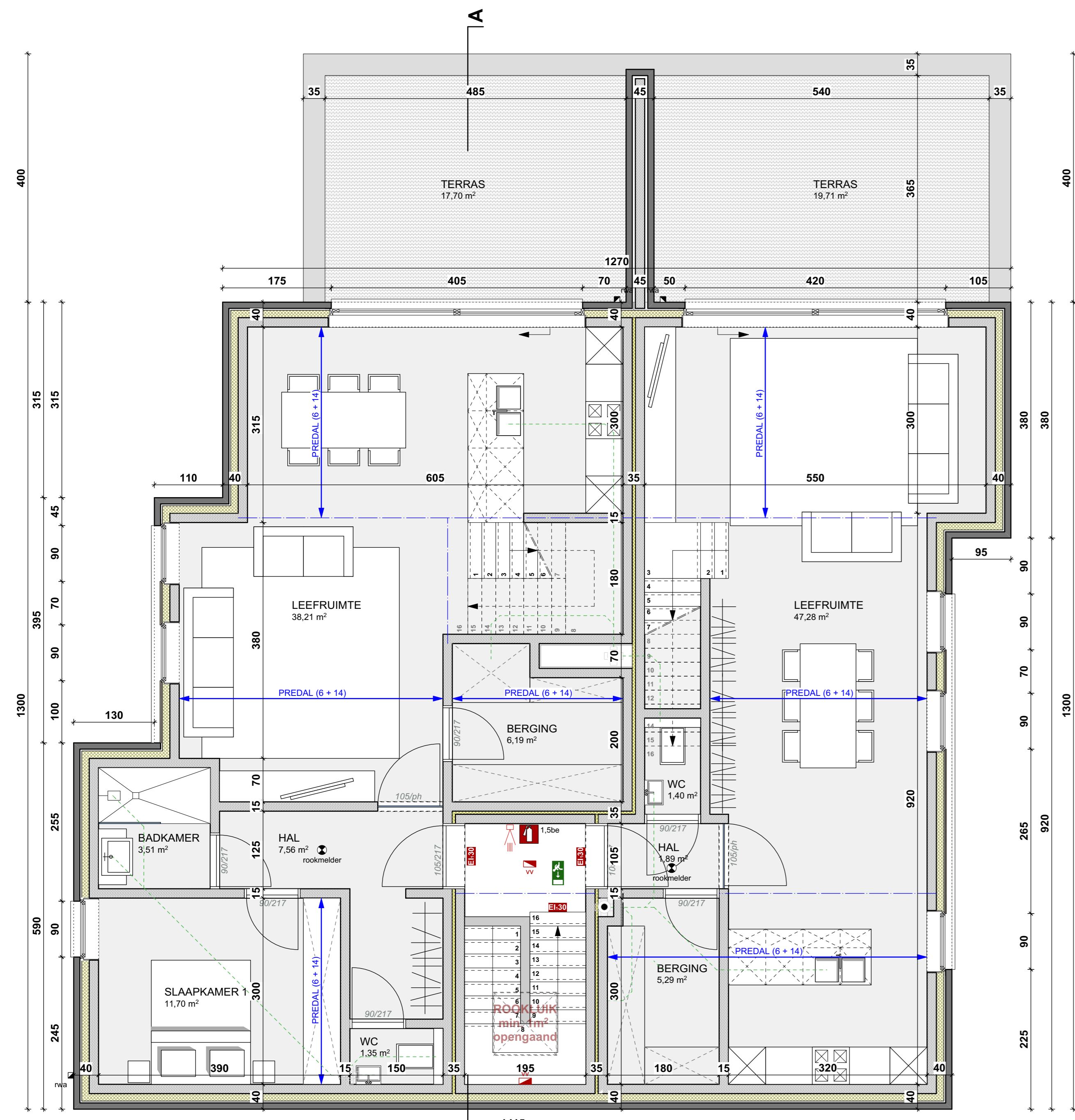
VERDIEPING 1 BLOK A schaal 1/50
