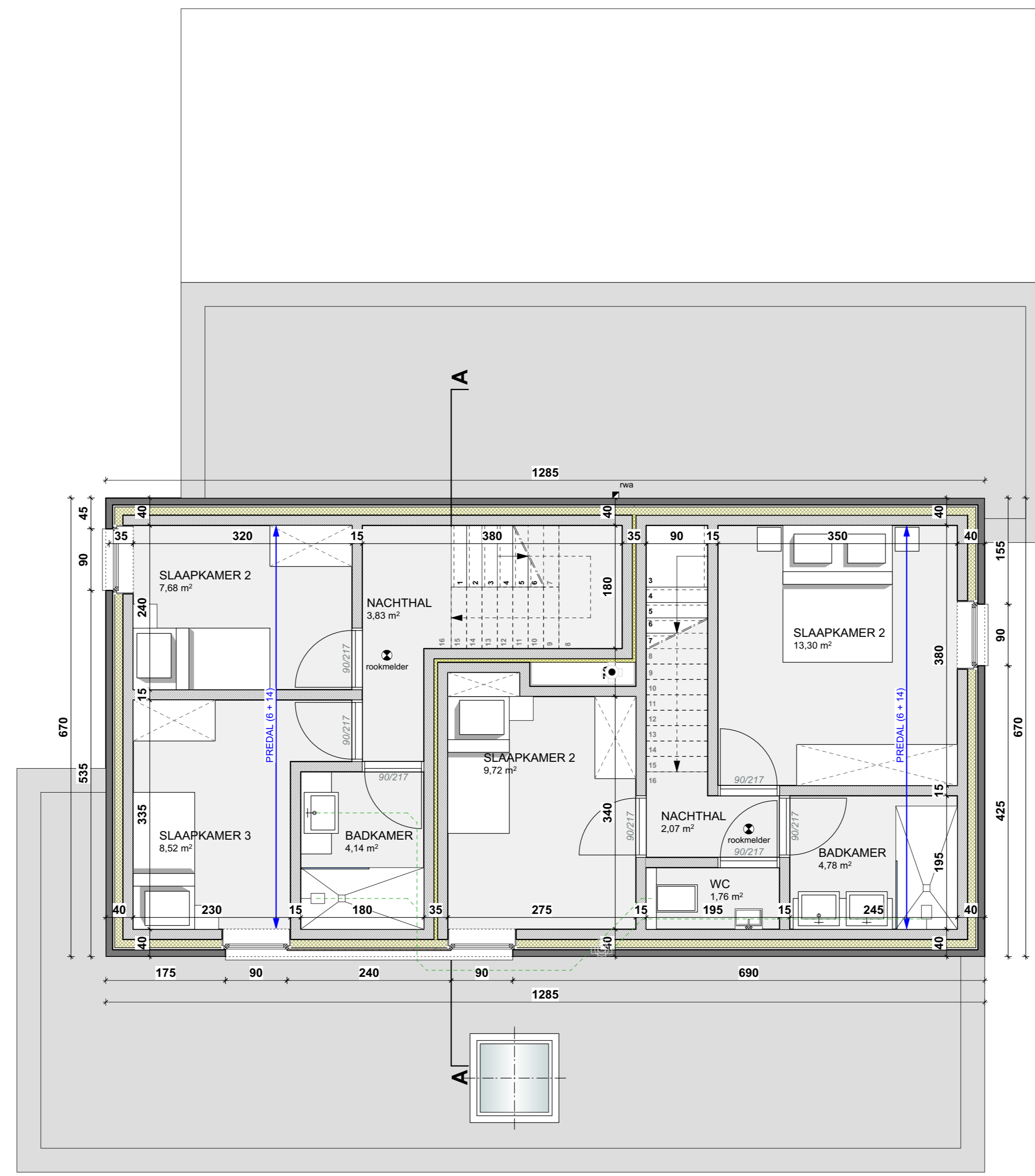
VERDIEPING 2 BLOK B schaal 1/50
