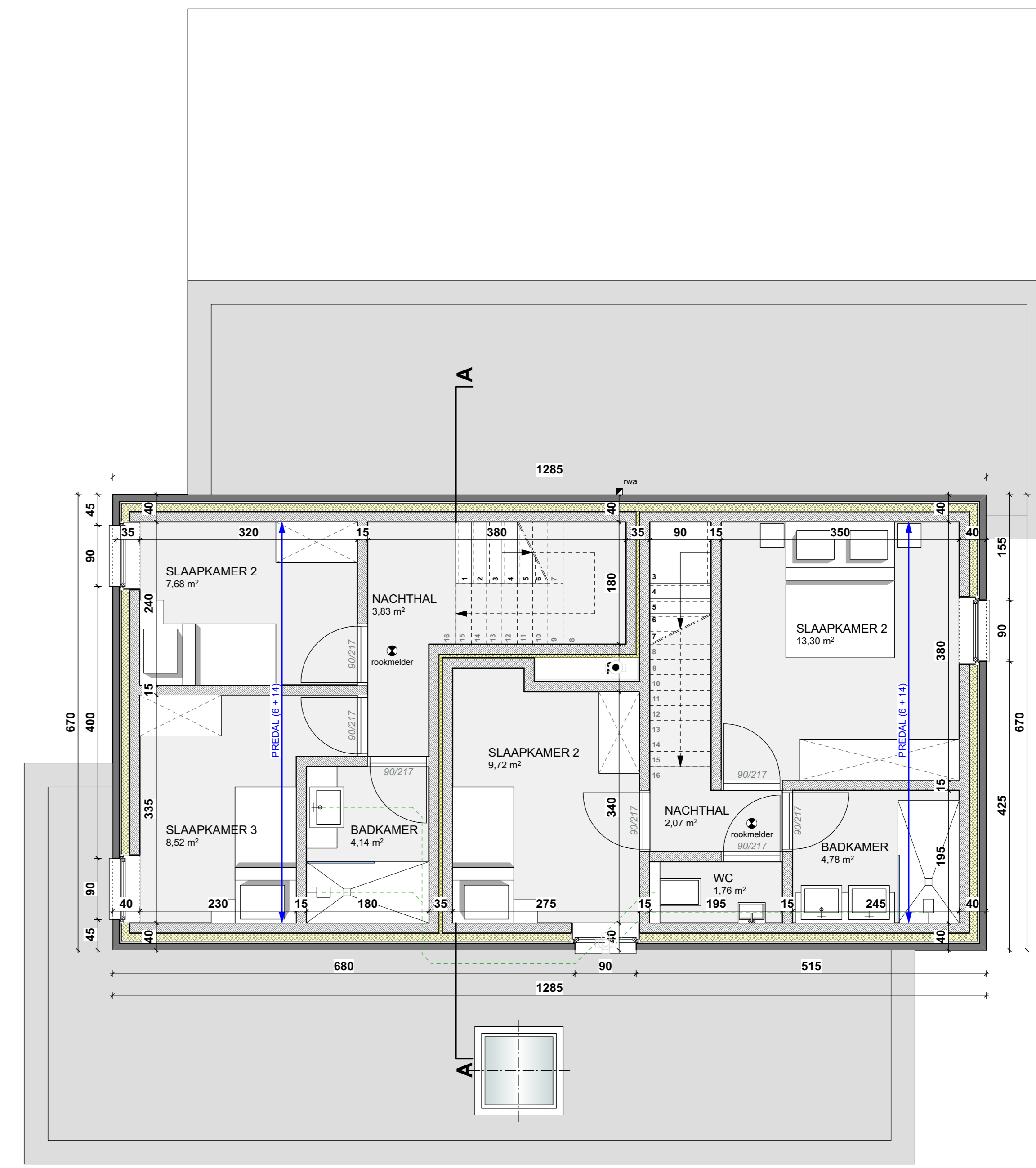
VERDIEPING 2 BLOK C schaal 1/50
