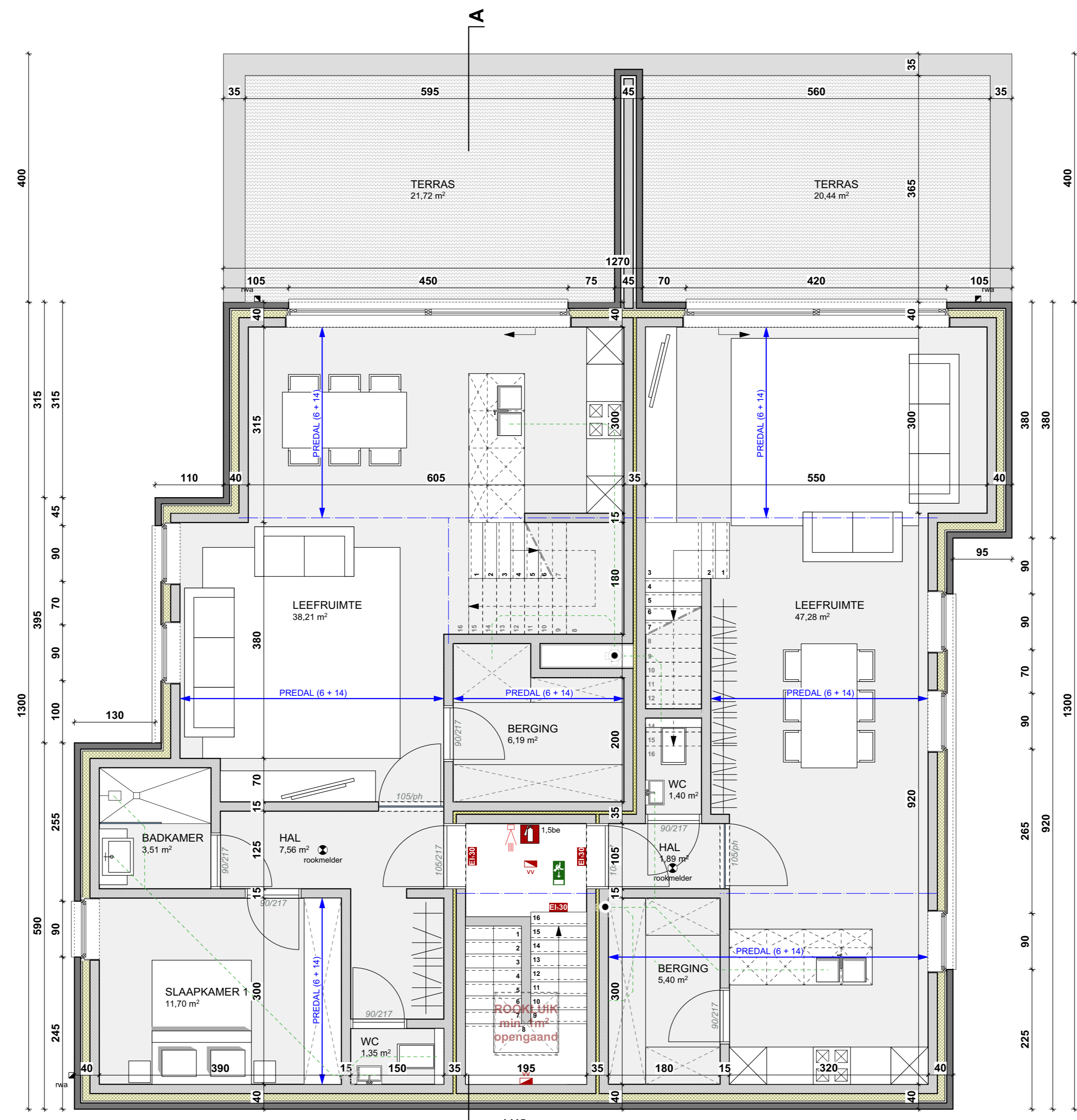
VERDIEPING 1 BLOK B schaal 1/50
