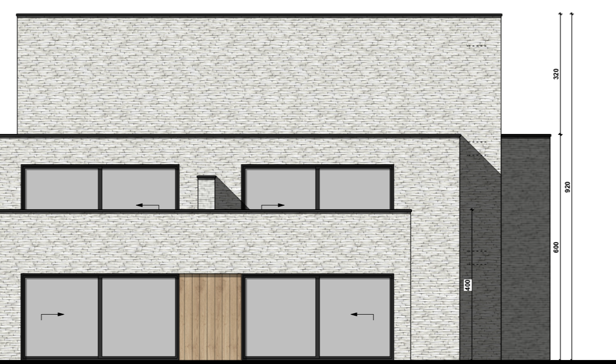
ACHTERGEVEL BLOK A schaal 1/100
