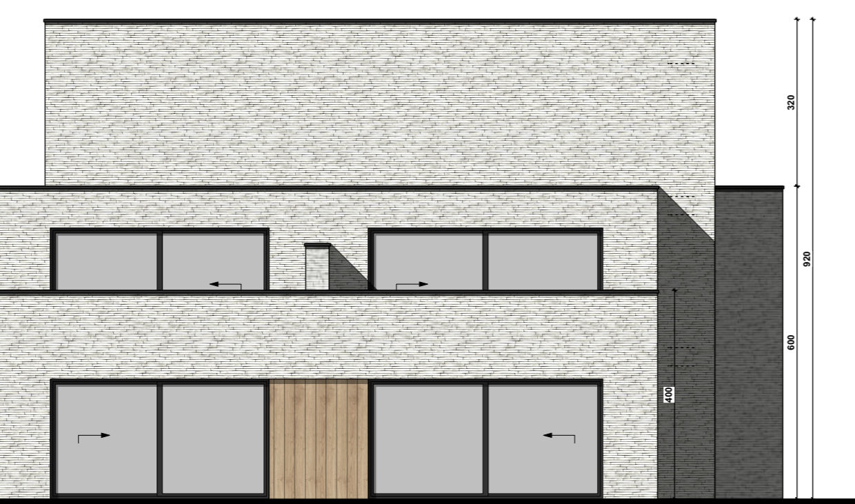
ACHTERGEVEL BLOK B schaal 1/100
