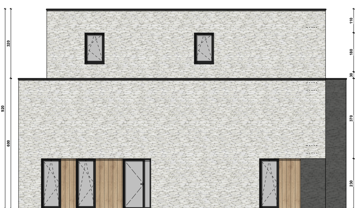
VOORGEVEL BLOK A schaal 1/100
