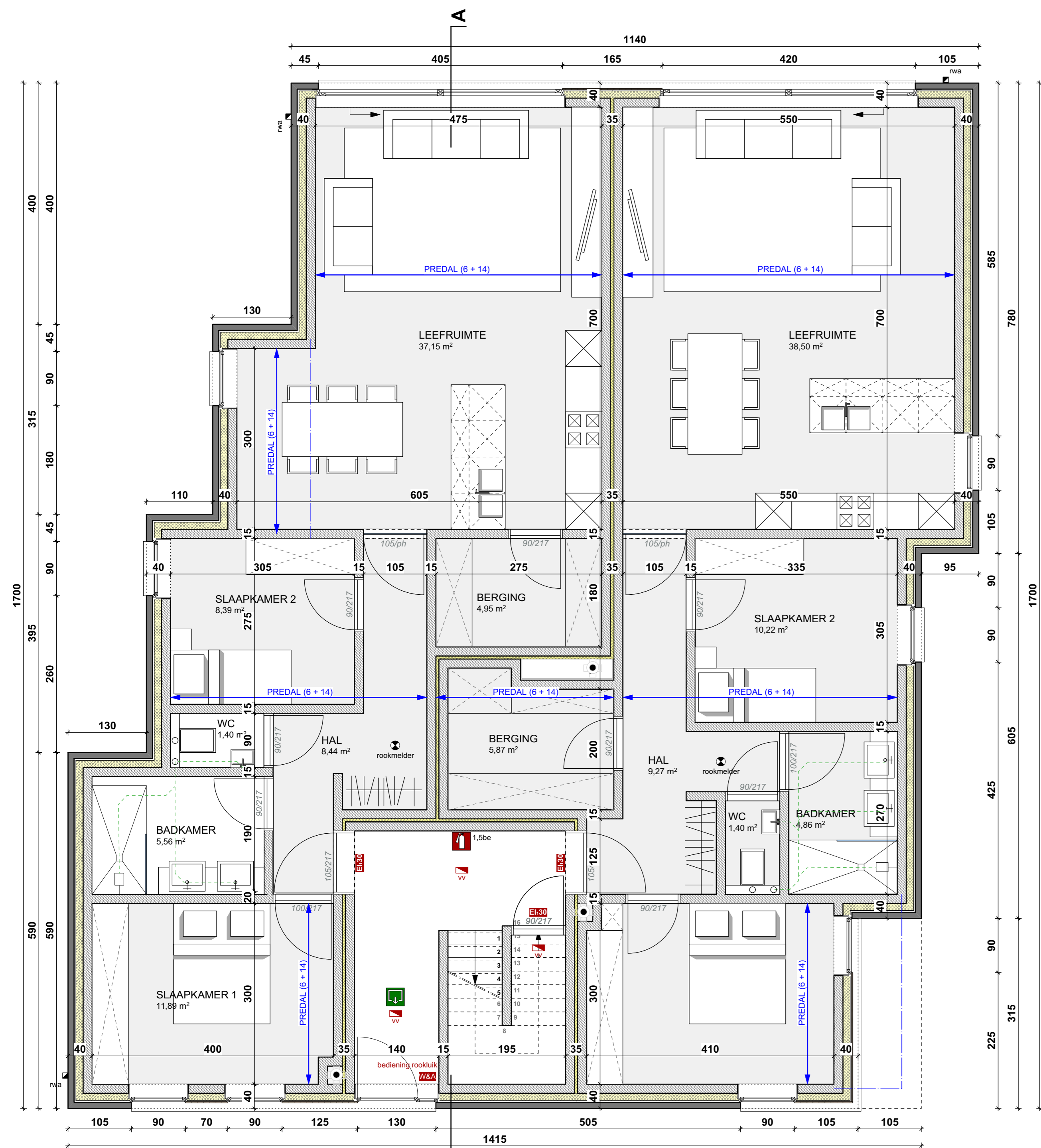
GELIJKVLOERS BLOK A schaal 1/50
