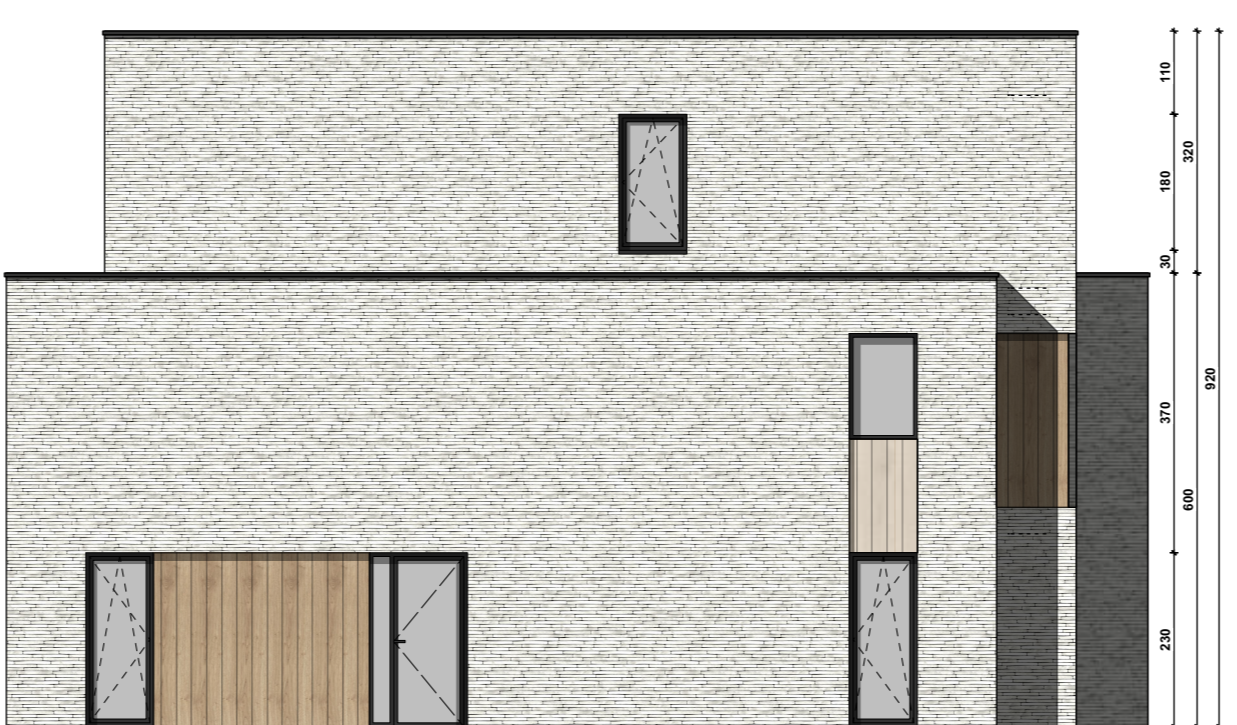
VOORGEVEL BLOK C schaal 1/100
