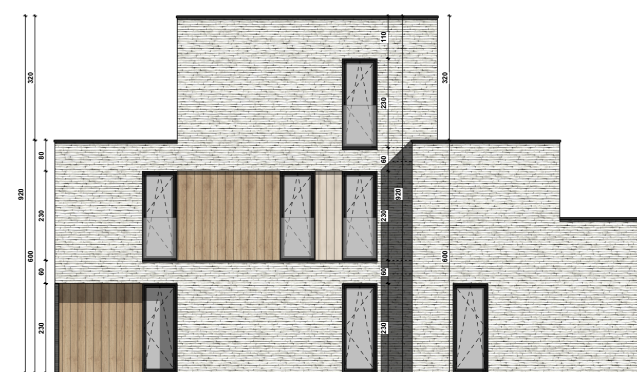
ZIJGEVEL RECHTS BLOK A schaal 1/100
