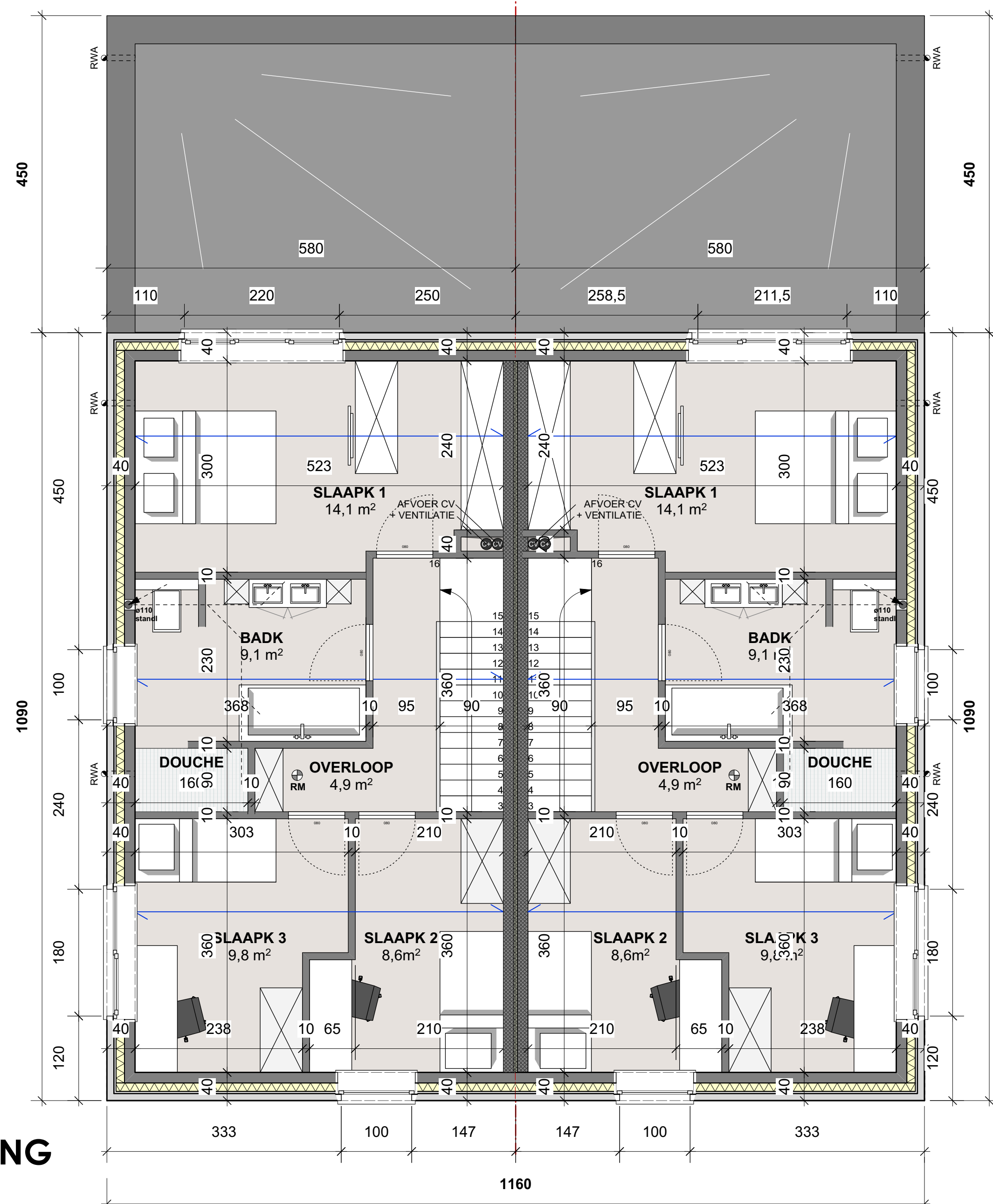
GELIJKVLOERS schaal 1/50
